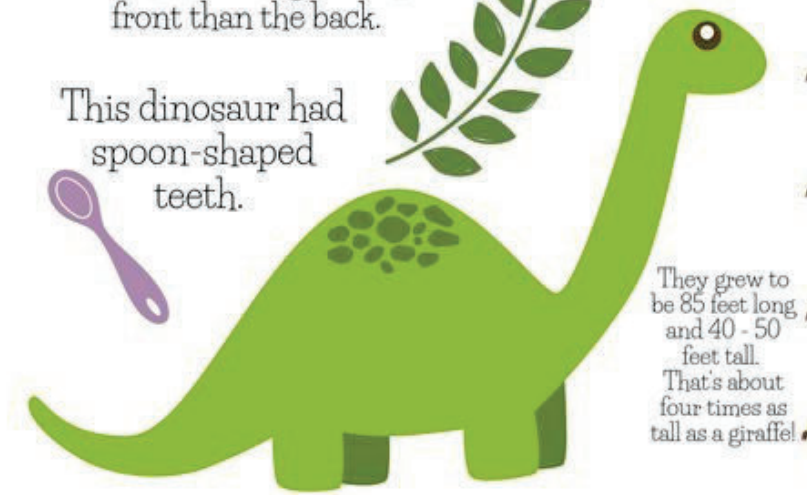
Brachiosaurus
