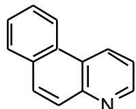
5,6-Benzoquinoline 5.15*
